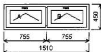
Dvojdielne okno s priečnikom
