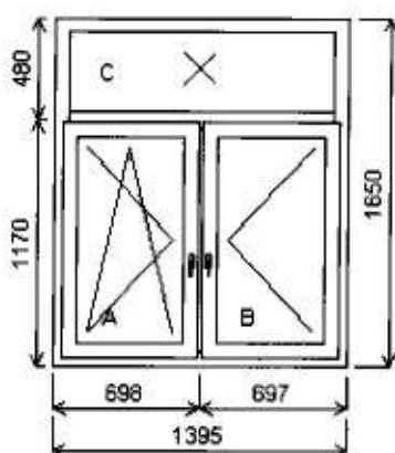
Trojdielne okno s nadsvetlíkom a priečnikom
