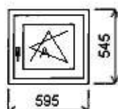
Jednodielne okno
